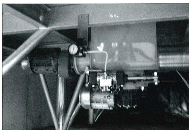
Zware bodemconstructie met aandrijfunit voor de uitdraagvijzel
